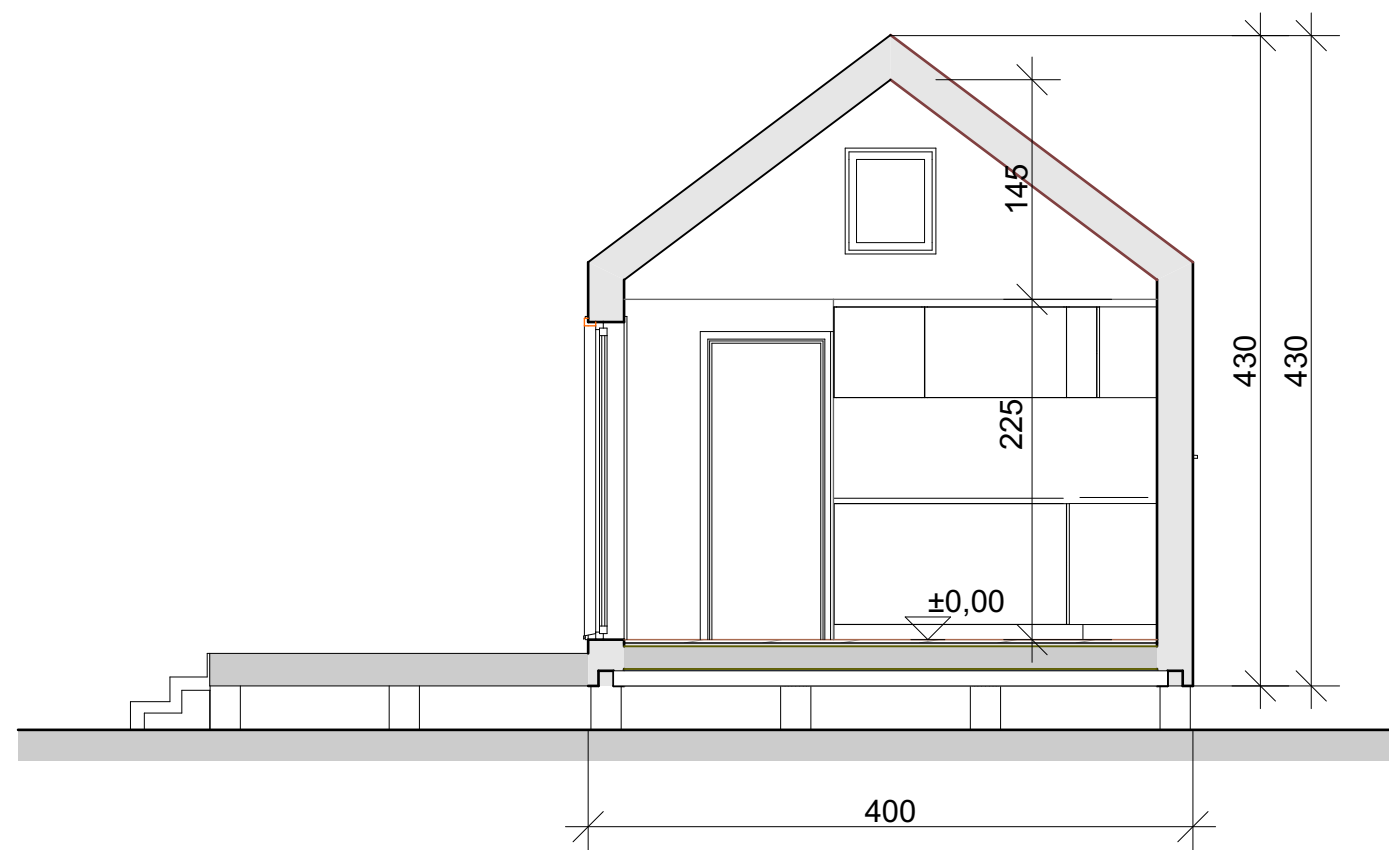
PJŪVIS 1-1 1:50
